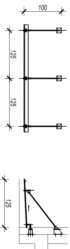
RYS. B DOTYCZY ZADASZENIA NA ELEWACJI "F"
